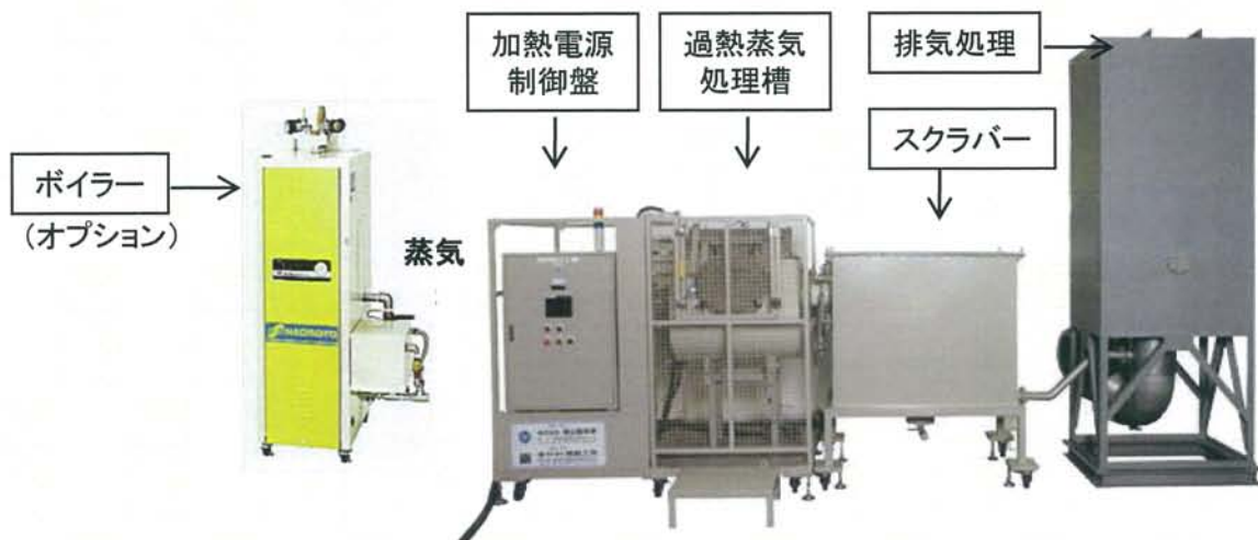
紙おむつ処理装置の外観
